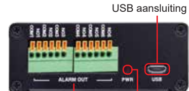
Alarm uitgangen Power led
